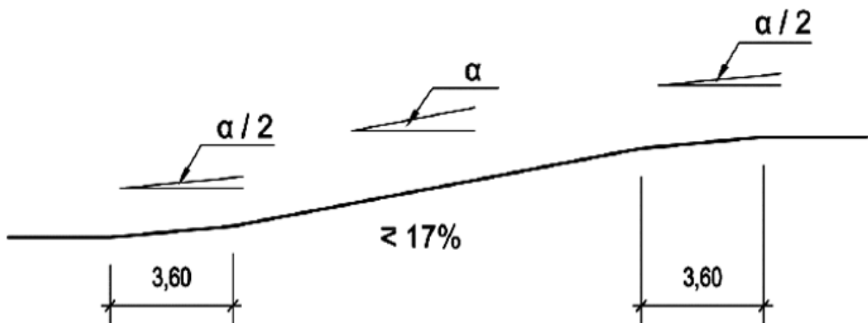
2. ábra: az álláshelyekhez vezető lejtő (közlekedési rámpa)
