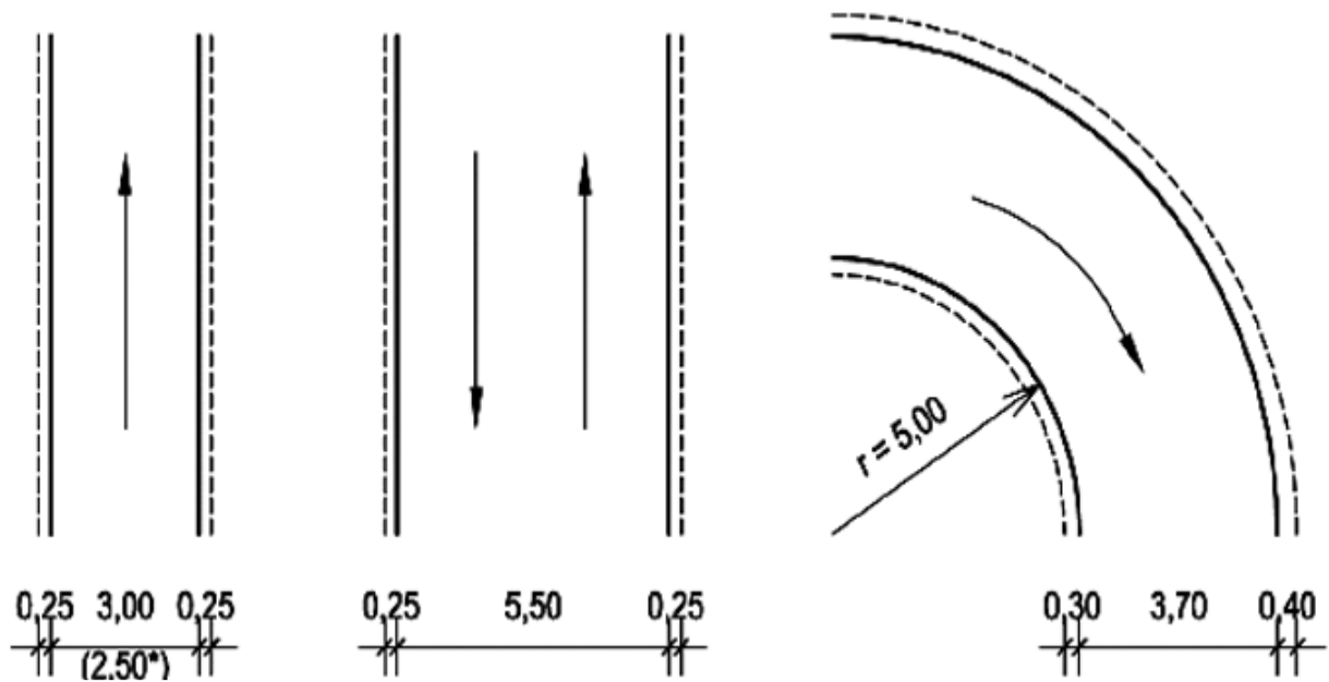
1. ábra: az álláshelyekhez vezető közlekedési út egyenes és íves szakaszai (rendszeres gyalogosforgalom nélkül)
